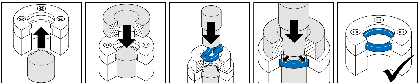
1B. Fitting with Pusher, cone sleeve and stops | Montage avec mandrin, douille conique et contre-appui | Construido con Pusher, manga cono y paras | Construído com Pusher, cone manga e batente
