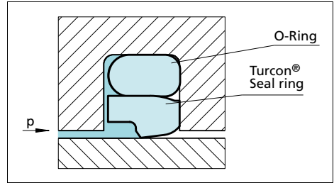
Figure 15 Turcon® Stepseal® 2K
